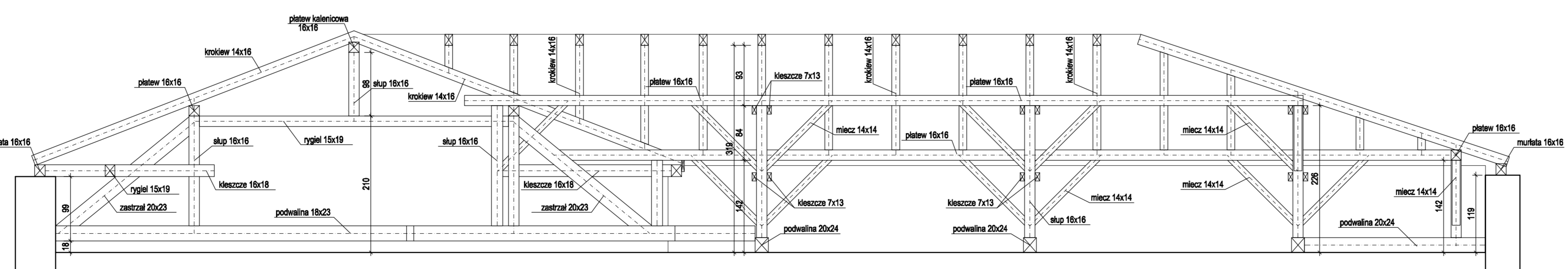
PRZEKRÓJ C-C
